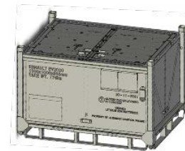
그림: 회수용 팩 포장 사양
